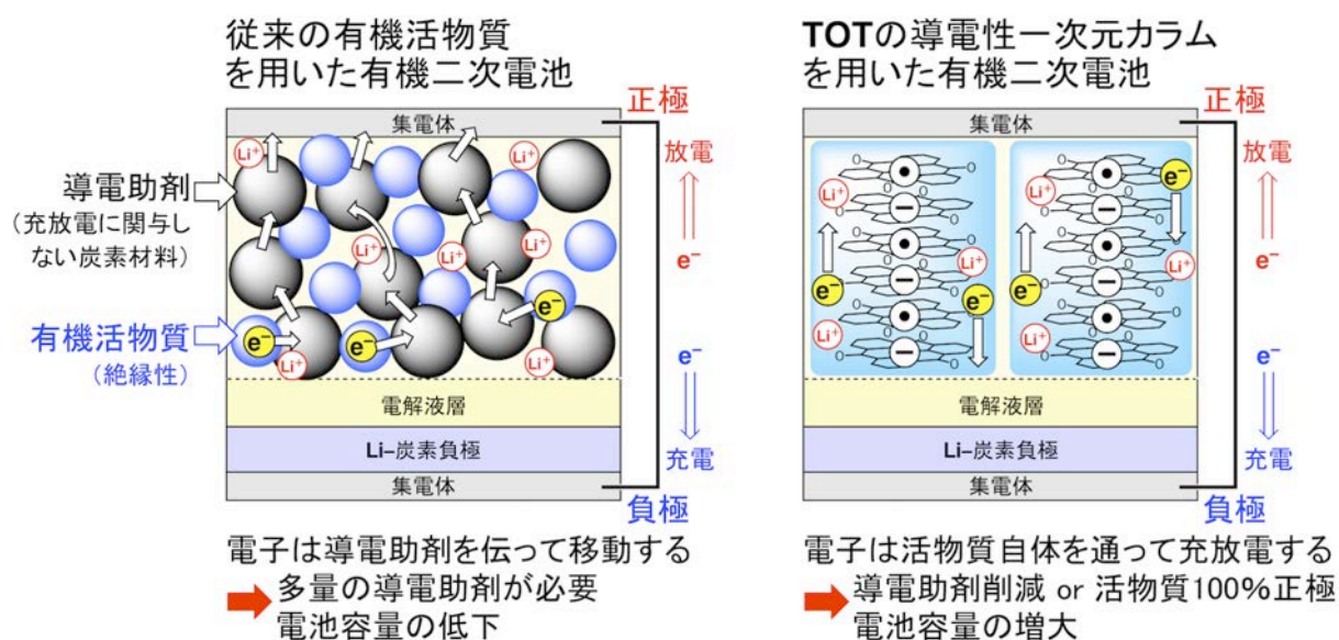
図8. 通常の有機活物質を用いたリチウムイオン二次電池(左)と導電性一次元 \pi 積層カラム構造を持つTOTを用いたリチウムイオン二次電池における正極中での電子移動経路の模式図。通常の有機分子は絶縁体で電気をほとんど流さないため、電極全体に電子を行き渡らせて活物質すべてを充放電させるには大量の導電助剤(アセチレンブラックやカーボン繊維などの炭素材料)が必要となる。多くの場合は、正極中の導電助剤の割合が90 wt%程度であり、充放電に関与できる活物質の割合が相対的に少なくなってしまうために、活物質あたりの容量を大きくしても電池全体としての容量は小さくなってしまいう傾向にある。一方TOT中性ラジカルは、一次元 \pi 積層カラム内を電子が移動できるため、現行の二次電池の正極活物質であるコバルト酸化物( \sigma_{RT} \sim 10^{-2} \text{ S cm}^{-1} )と同等あるいは若干低い程度の電気伝導性を示す。特に充放電途中の状態である混合原子価状態ではさらに高い電気伝導性を示すため、導電助剤の量を大幅に削減あるいは全く含まない条件での充放電が可能になると考えられる。現在、これらのことに着目した有機二次電池の改良についての研究を展開しており、「有機活物質を80 wt%以上含む正極」や上述の「TOT中性ラジカルの真空蒸着高配向性薄膜による有機活物質100%の正極」を用いたリチウムイオン二次電池など、従来の有機活物質では実現不可能な二次電池デバイスの研究開発を進めています。
