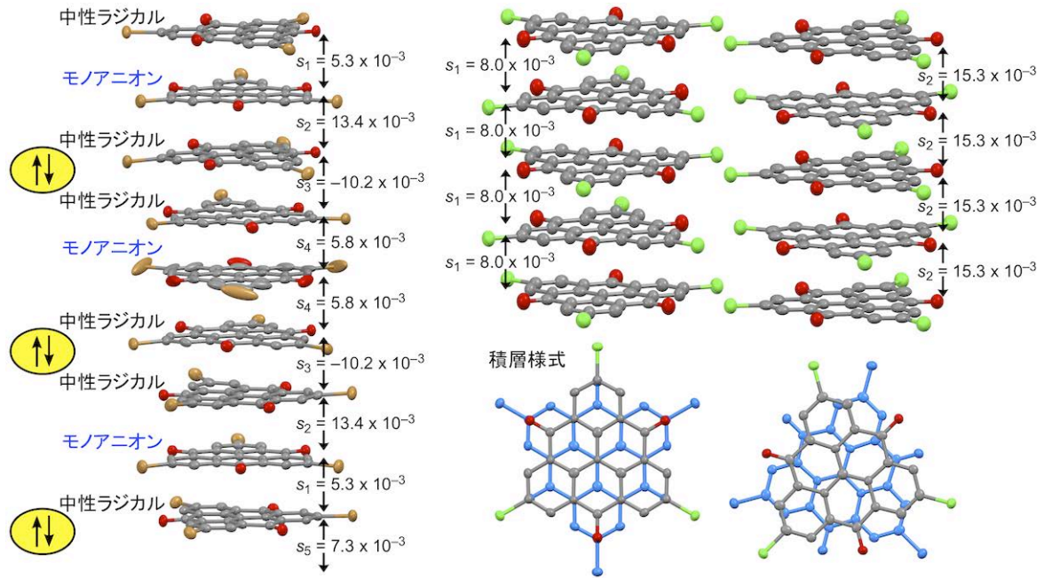
図7. \text{Br}_3\text{TOT} の混合原子価塩 ( n\text{-Bu}_4\text{N}^+ ) ( \text{Br}_3\text{TOT}^- ) ( \text{Br}_3\text{TOT} ) 2 (左) および \text{Cl}_3\text{TOT} の混合原子価塩 \text{Li}^+ ( \text{Cl}_3\text{TOT}^- ) ( \text{Cl}_3\text{TOT} ) x の一次元 \pi 積層カラム構造と重なり様式 (右)。いずれの塩でも中性ラジカルの一次元 \pi 積層カラムにモノアニオン種が注入されたことで、飛躍的な電気伝導性の向上が見られた。 \text{Br}_3\text{TOT} 塩では中性ラジカルとモノアニオン種がカラム内で2 : 1の割合で規則正しく配列している様子が詳細なX線結晶構造解析からわかった。この時、積層内で中性ラジカルが2つ並んだ部分で反強磁性的な相互作用が働いていると思われる。一方、 \text{Cl}_3\text{TOT} のリチウム塩では、結晶構造中に2種類の積層のカラム構造が形成されていた。いずれのカラムにおいても、全ての \text{Cl}_3\text{TOT} 分子は等価、すなわち同じ電子状態を持つ分子として解析され、その積層面間距離と相互作用は均一であった。このことは、 \pi 積層カラム内を伝導電子が自由に移動できることを示唆しており、実際にこの塩は \text{Br}_3\text{TOT} 塩よりもさらに高い電気伝導性を示した。
