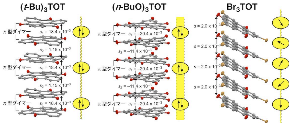
図5. (t\text{-Bu})_3\text{TOT} , (n\text{-BuO})_3\text{TOT} , \text{Br}_3\text{TOT} 中性ラジカル的一次元 \pi 積層カラム構造 ( \pi 積層ラジカルポリマー)。分子間の相互作用の強さを「重なり積分 ( s )」で示している。黄色の楕円と矢印は、分子間相互作用と電子スピンの配向性を模式的に示したもの。 (t\text{-Bu})_3\text{TOT} では \pi 型ダイマー内の相互作用( s_1 )に比べて、 \pi 型ダイマー間の相互作用( s_2 )の大きさが1/16と非常に小さい。 \pi 型ダイマー内の2個の不对電子は電子スピンを反対向きにして強固な対を形成し(反強磁性的相互作用、図中矢印)、 \pi 型ダイマー内に閉じ込められたため、この結晶は絶縁体になった。 (n\text{-BuO})_3\text{TOT} も同様に \pi 型ダイマーが積層して一次元 \pi 積層カラム構造を形成しているが、 \pi 型ダイマー間の相互作用 s_2 が (t\text{-Bu})_3\text{TOT} の場合と比べて10倍近く大きく、 \pi 型ダイマー内の相互作用 s_1 と拮抗している。そのため、 \pi 型ダイマー内の反強磁性的相互作用による閉じ込め効果が弱く、高い電気伝導性を示した。 \text{Br}_3\text{TOT} は \pi 型ダイマーを形成せず、全ての積層距離・相互作用が同じ均一な \pi 積層カラム構造を形成している。面間距離が他と比べて若干大きいために相互作用 ( s ) 自体は小さいものの、 \pi 型ダイマー化による閉じ込め効果がなく、電子スピンは比較的自由的な配向をとる。そのため、電子は比較的自由に移動でき高い電気伝導性を示した。
